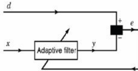
شکل (۱): ساختار کلی فیلتر وقتی
