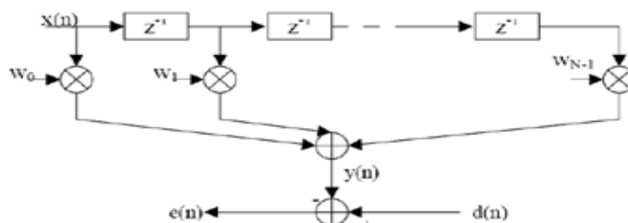
شکل (۲): فرآیند الگوریتم LMS و فیلترینگ عرضی
