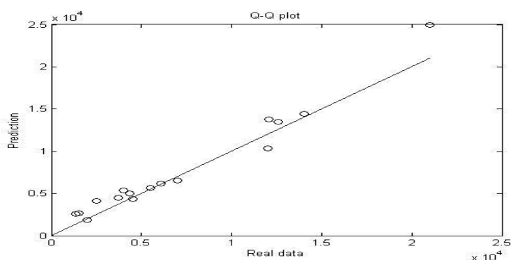
نمودار ۴- پراکندگی داده های واقعی و داده های پیش بینی مدل شبکه عصبی
